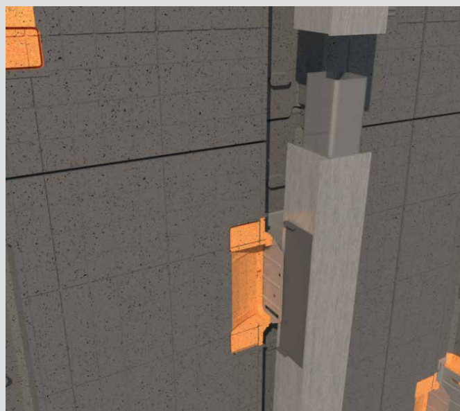
Profielen onderling verbinden met profielverbinder. De korte profielen werken nu als één lang profiel en is daardoor eenvoudig waterpas te stellen.
