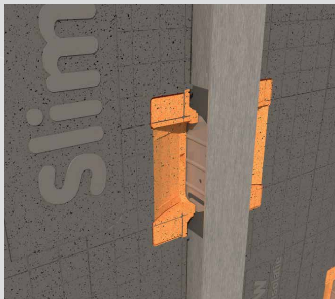
Profiel zit in bracket. Het nokje zit in slobgat. Eruit vallen is niet meer mogelijk. Nu is het profiel over een diepte van 23 mm te stellen.
